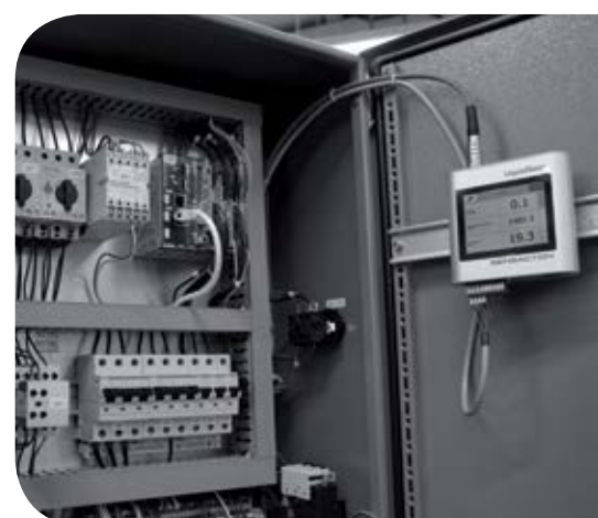
Bild oben: LiquidSens Controller Touch im Schaltschrank einer Reinigungsanlage
